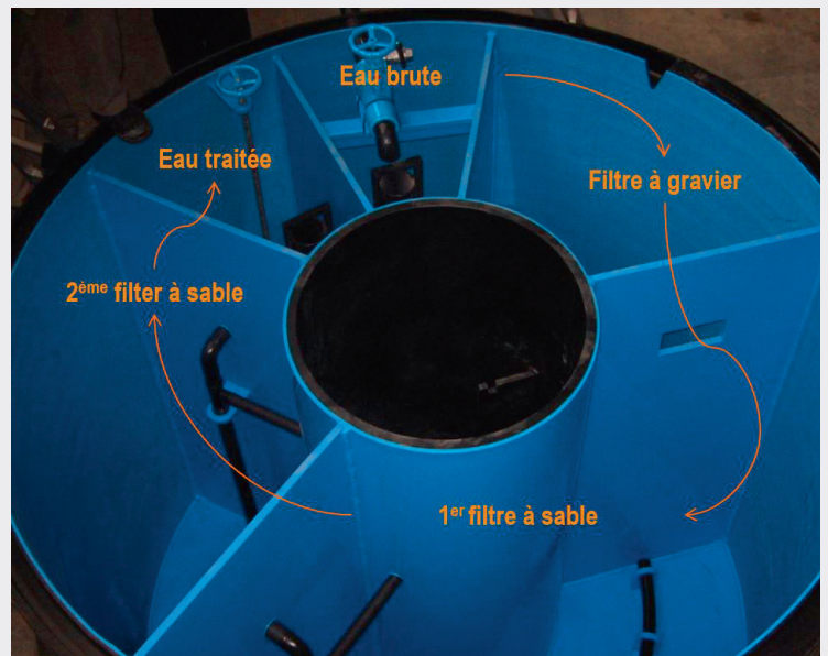
Fig. 3 Principe de fonctionnement du système de filtration
