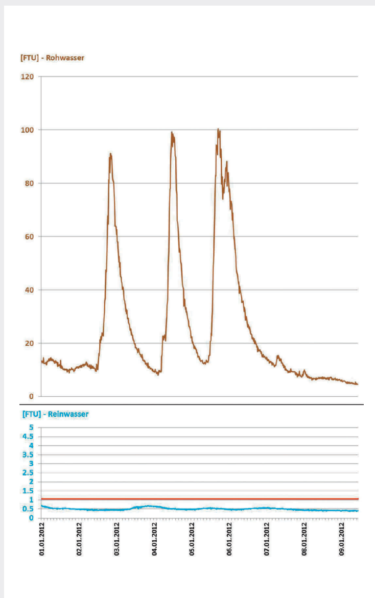
Fig. 5 Variation de la turbidité dans l'eau brute et traitée de l'installation pilote entre le 1 er et le 9 janvier 2012. Selon l'OSEC, la valeur de tolérance pour la turbidité est de 1 FTU
