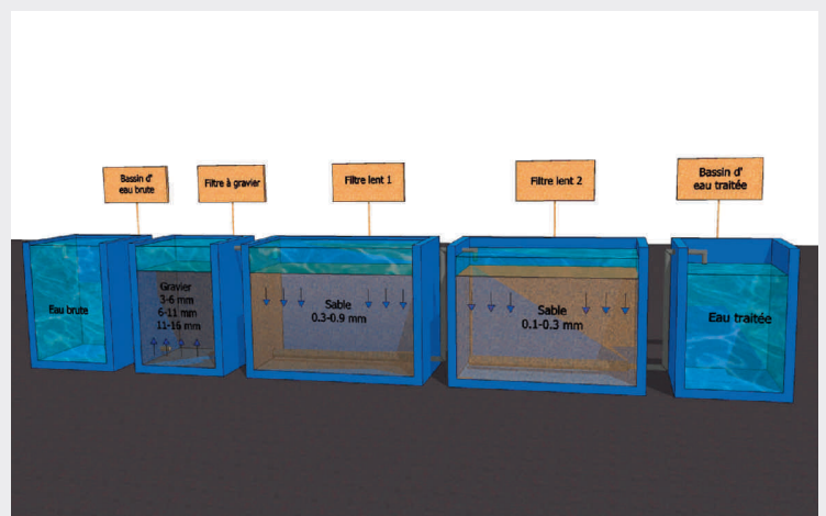
Fig. 4 Schéma d'écoulement du système de filtration
