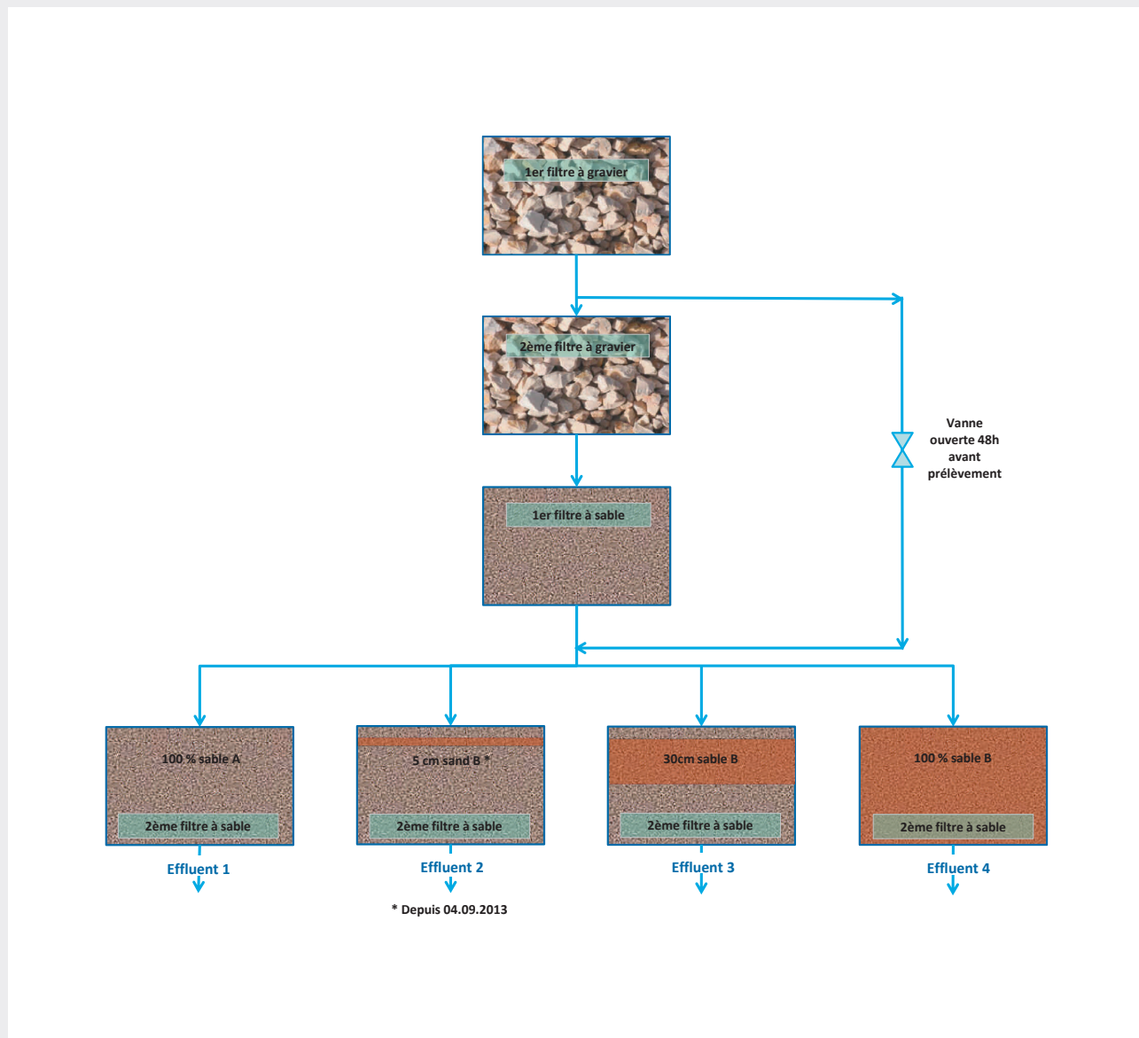
Fig. 6 Schéma de fonctionnement de l'installation pilote à Porrentruy JU Funktionsschema der Pilotanlage in Porrentruy JU
